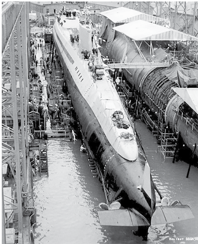
Tàu ngầm Halibut trên bệ đóng năm 1959
