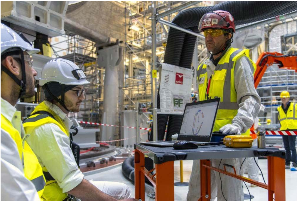
Các chuyên gia tập đoàn SIMANN (SIMIC-Ansaldo) đo đạc dữ liệu của bình hút chân không tại lò nhiệt hạch ITER (NGUỒN ẢNH: WWW.ITER.ORG)
