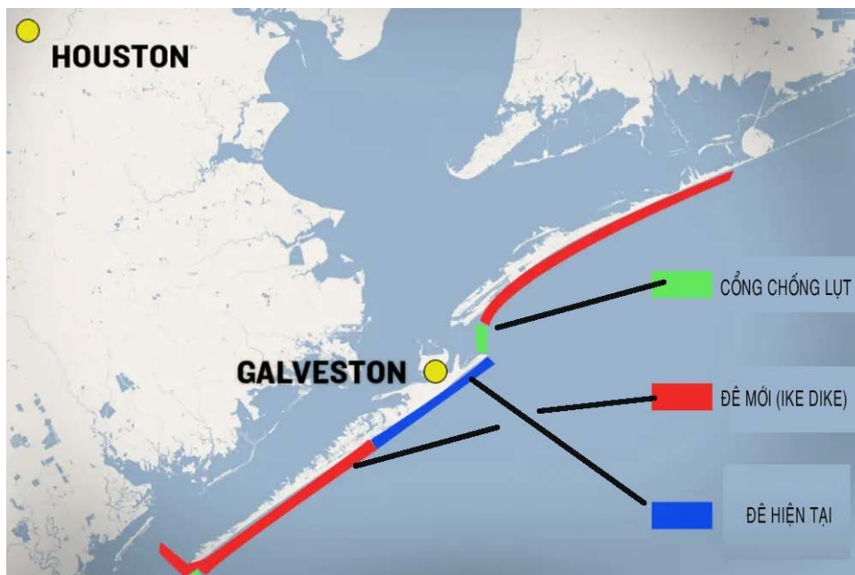
Sơ đồ công trình “Ike Dike”
