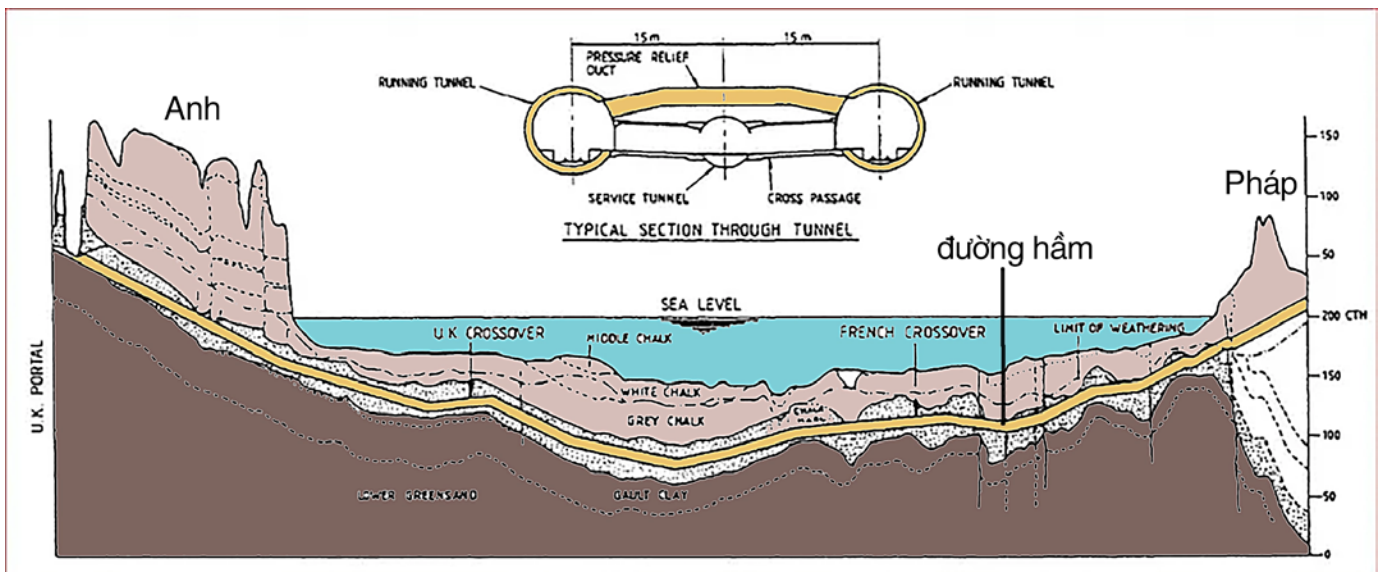
Sơ đồ đường hầm xuyên qua eo biển Manche, nối liền Anh và Pháp
